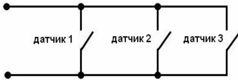
Схема 4.2. Тип шлейфа "на замыкание".
